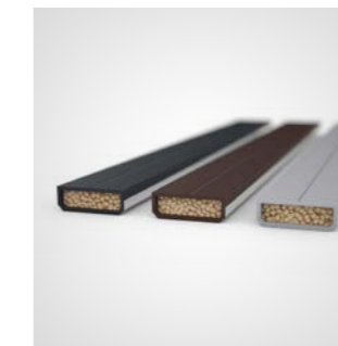
Canalina calda Swisspacer Ultimate (colori disponibili: nero, marrone, grigio).
